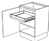
GOD1BL Onderkast 1 deur en 1 lade en 1 legplank.
